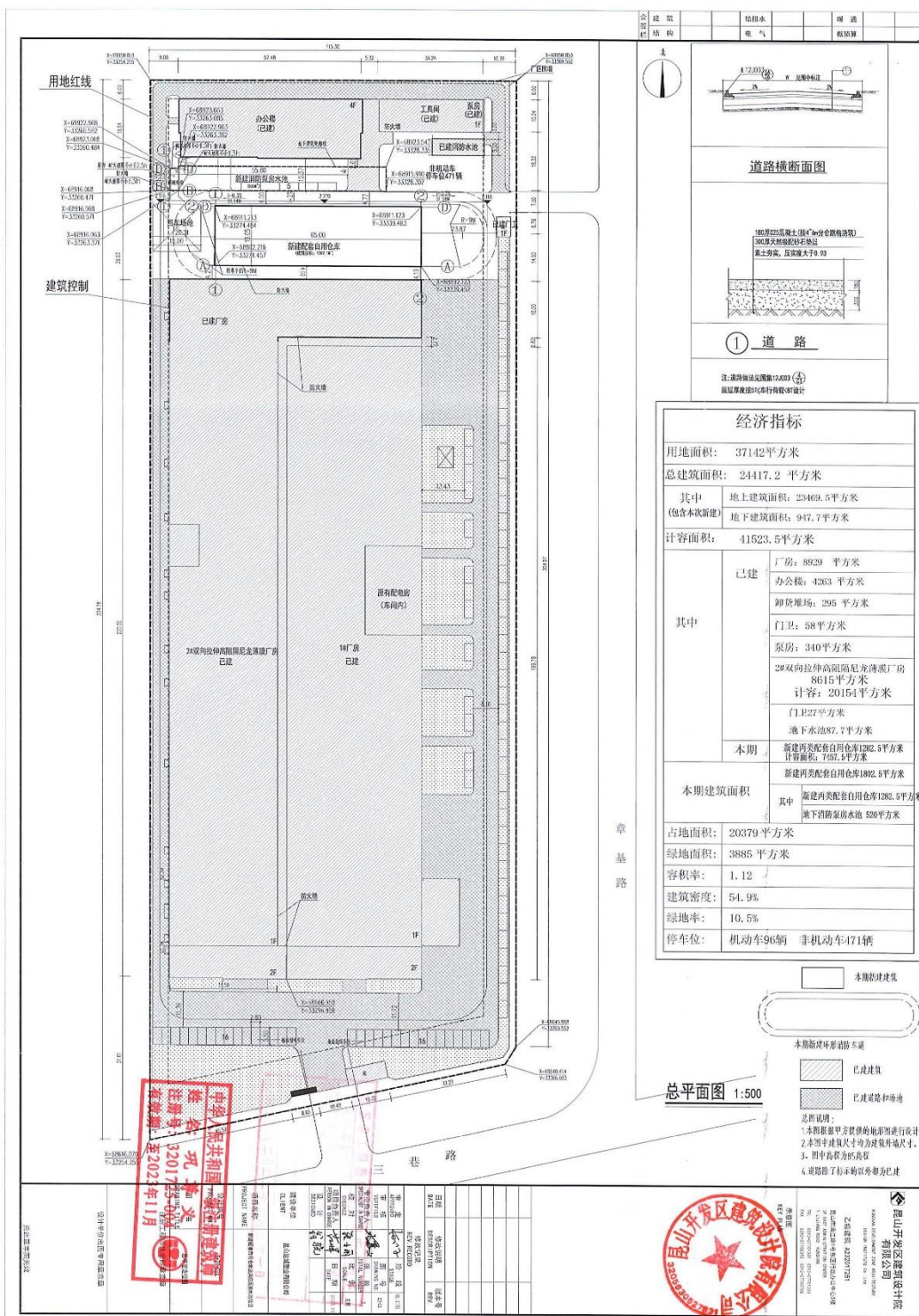
图 3.4 平面布局图
